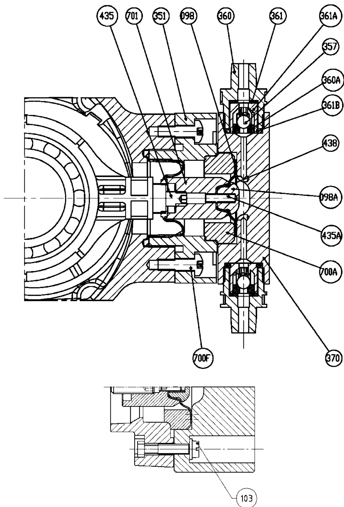
图5-5 GM0002~GM0010 PVC, PVDF液力端零件清单-螺纹连接
