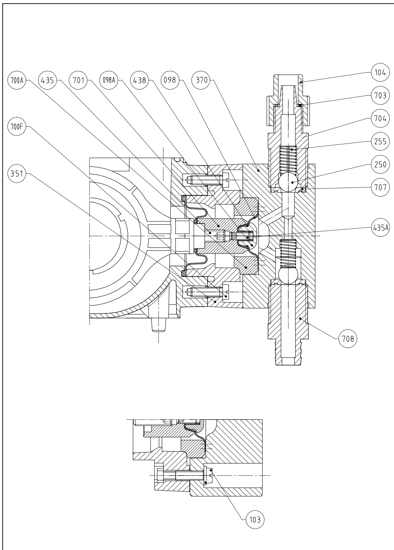
图5-7 GM0002~GM0010 高粘度液力端
