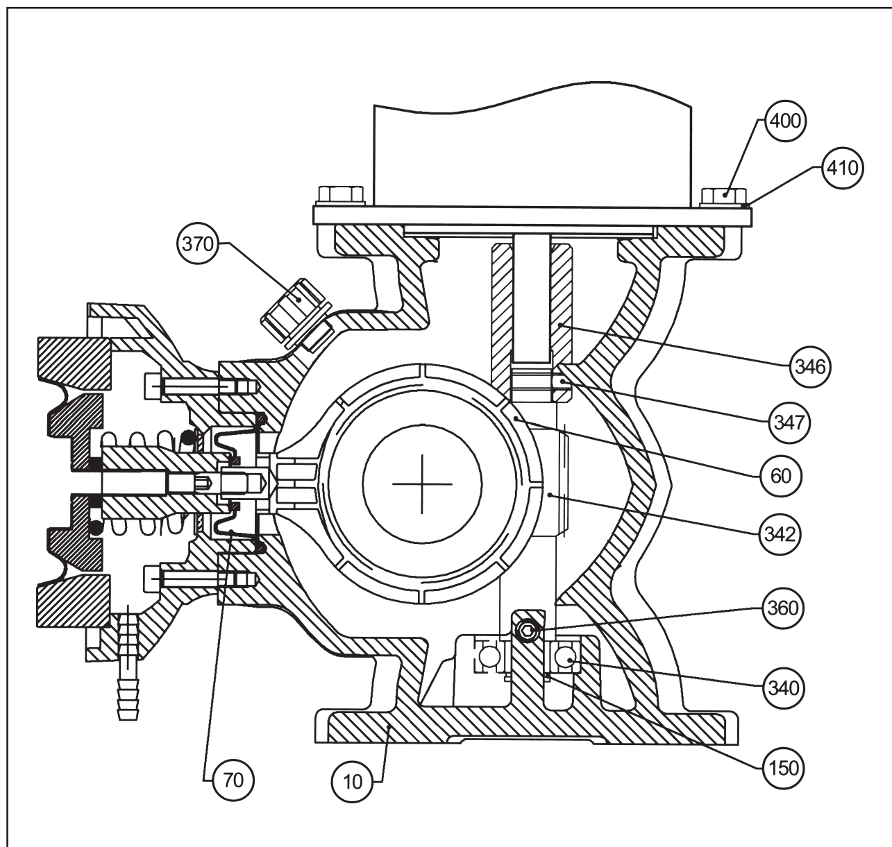
图5-1 GM 驱动端侧视图
