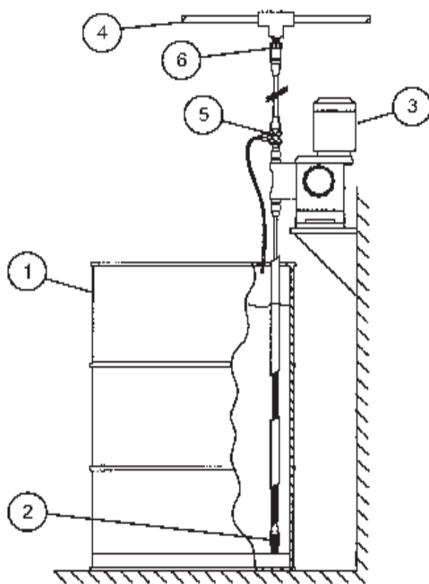
图2-2： 典型安装
