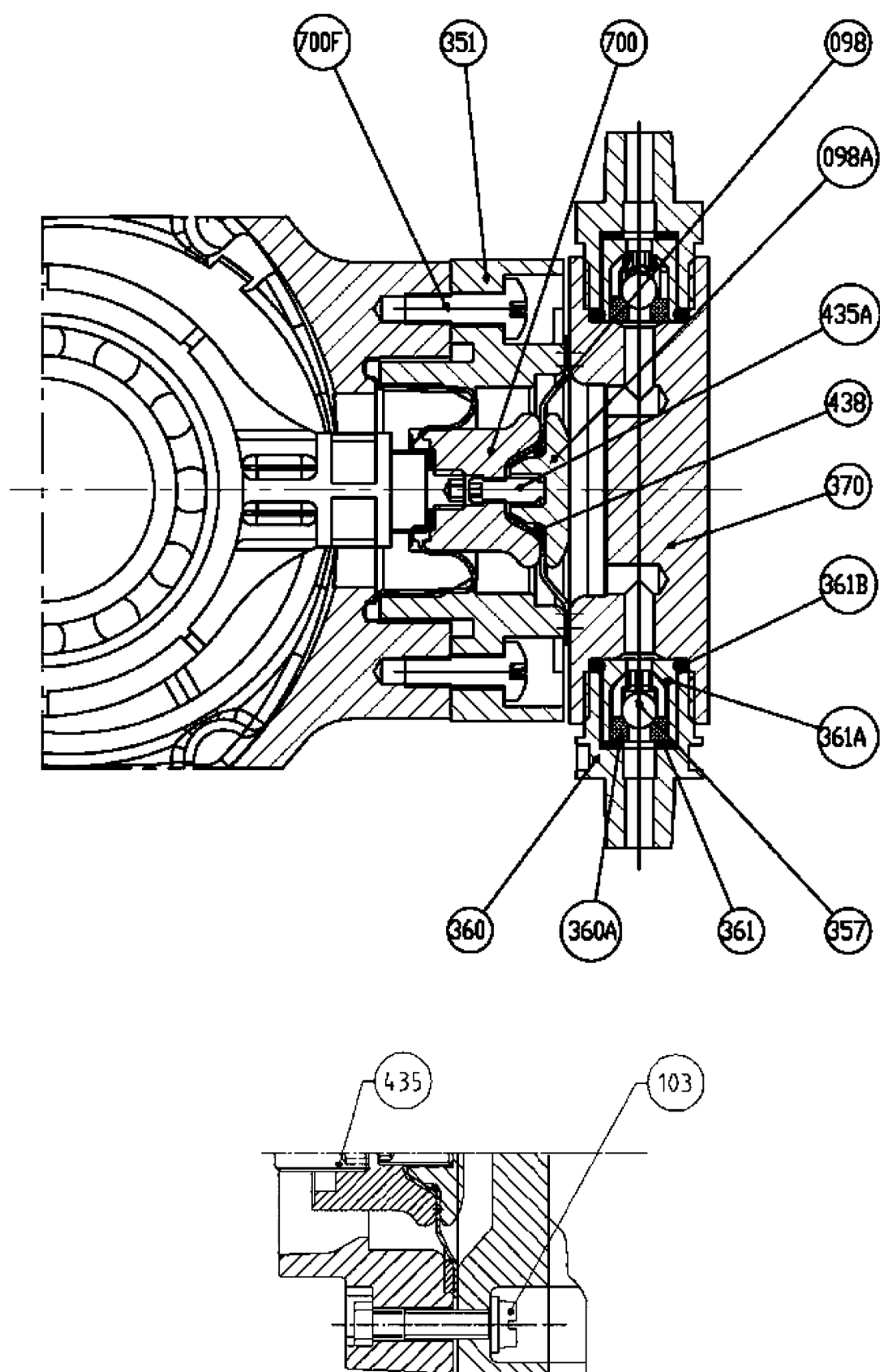
图5-10 GM0025~GM0050 PVC 液力端零件清单-螺纹连接
