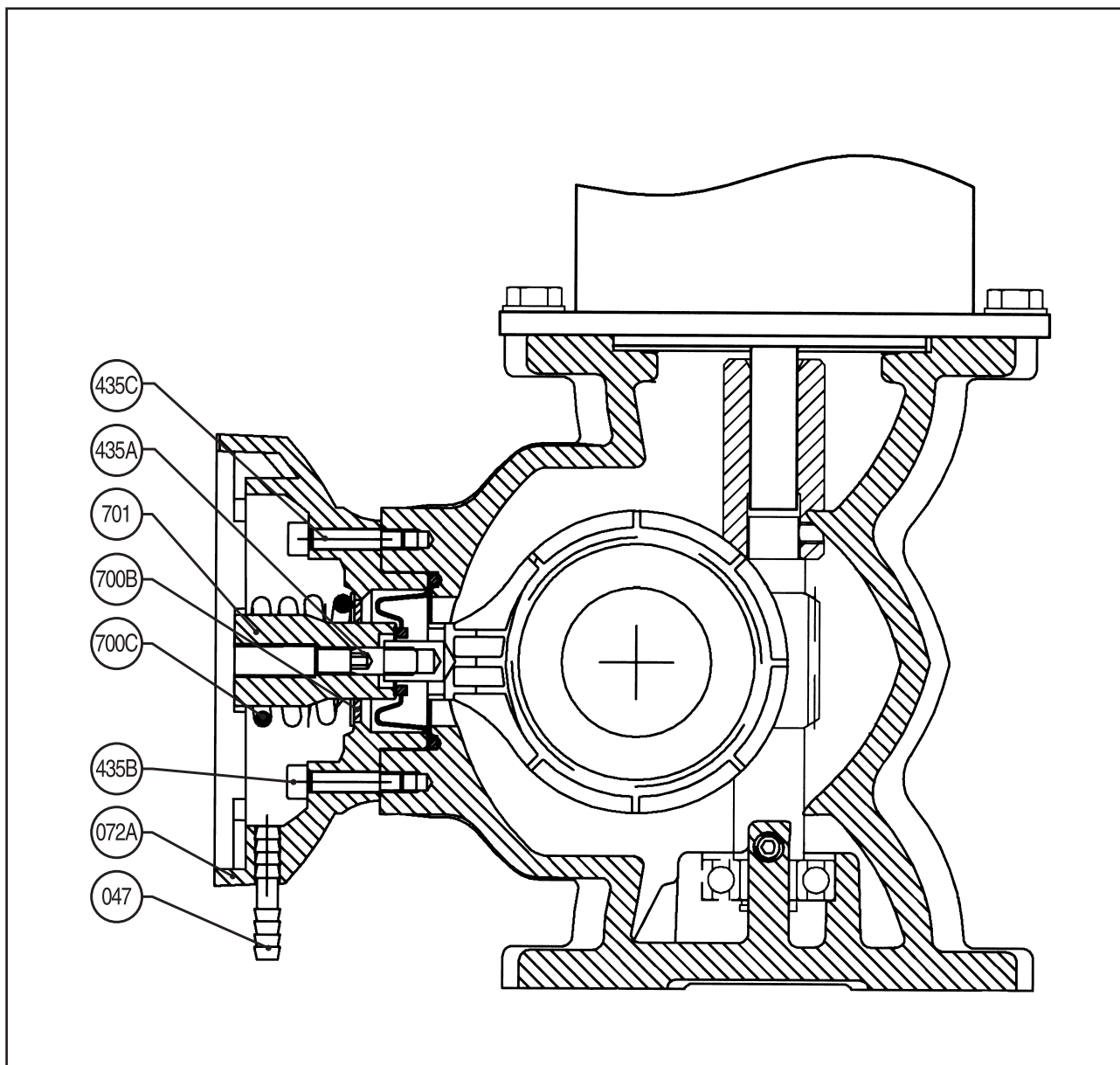
图5-13 GM0090~GM0500 中间段
