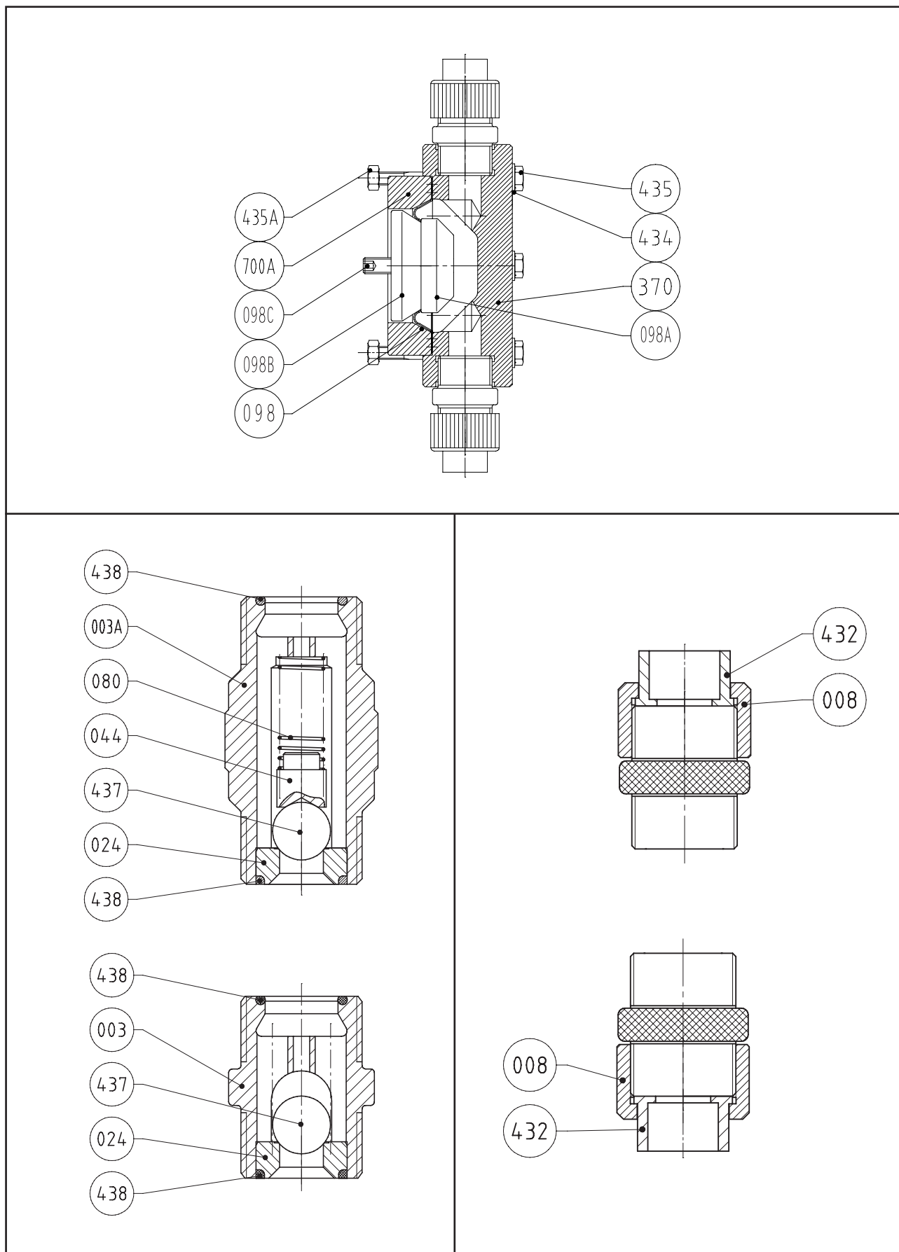
图5-16 GM0090~GM0500 高粘度液力端
