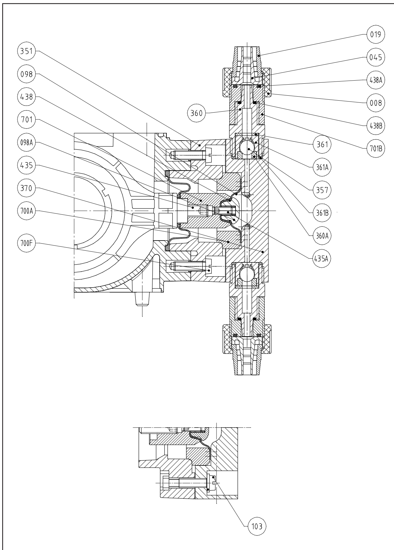
图5-3 GM0002~GM0010 PVC, PVDF & 混合物液力端
