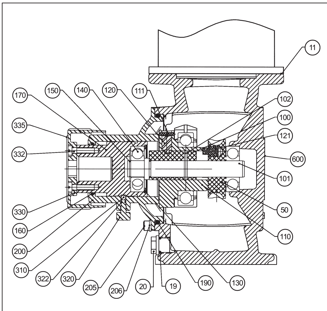
图5-2 GM 驱动端端面图
