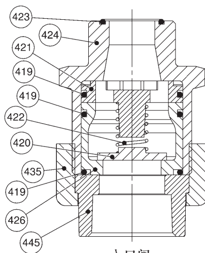
入口阀
