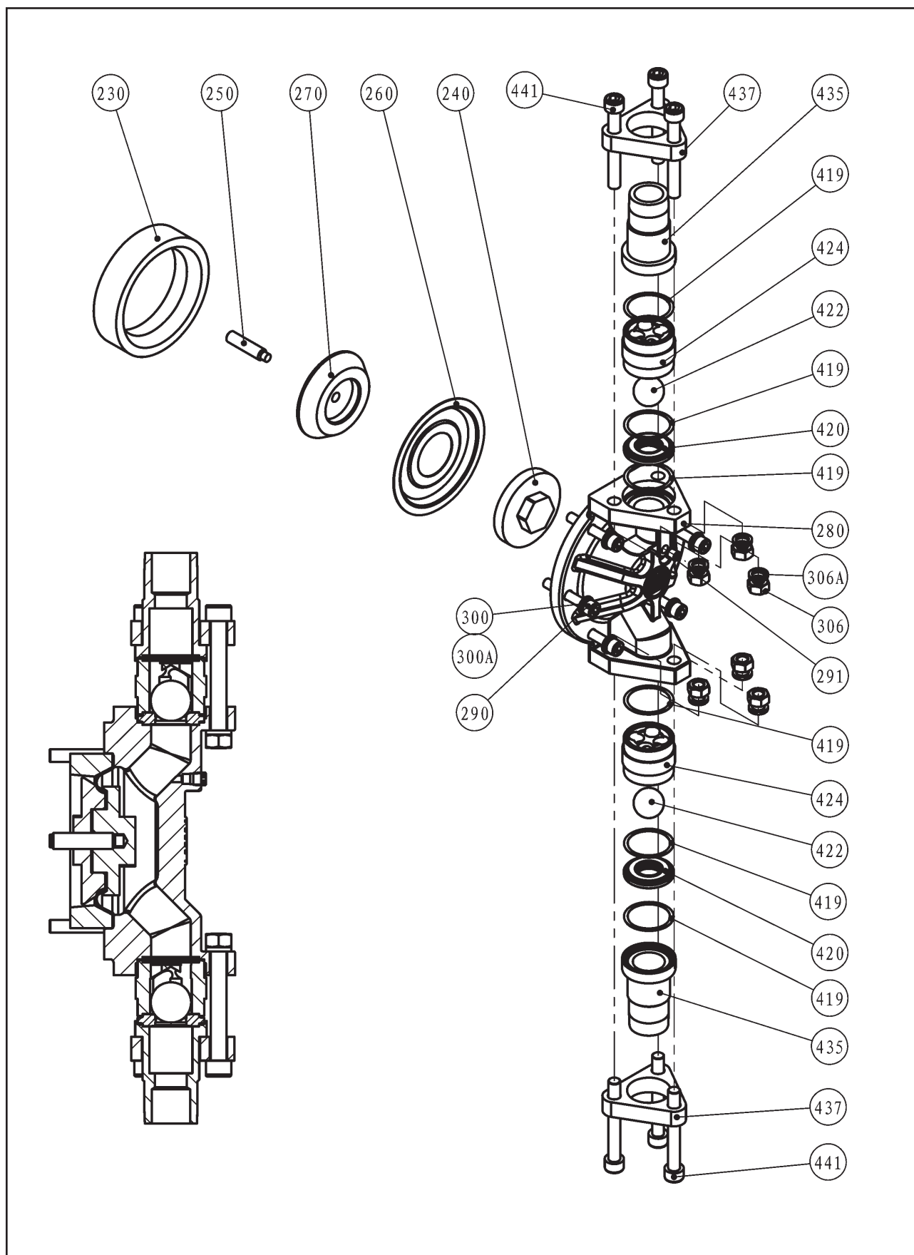
图6-13 GB0500~GB0600不锈钢液力端
