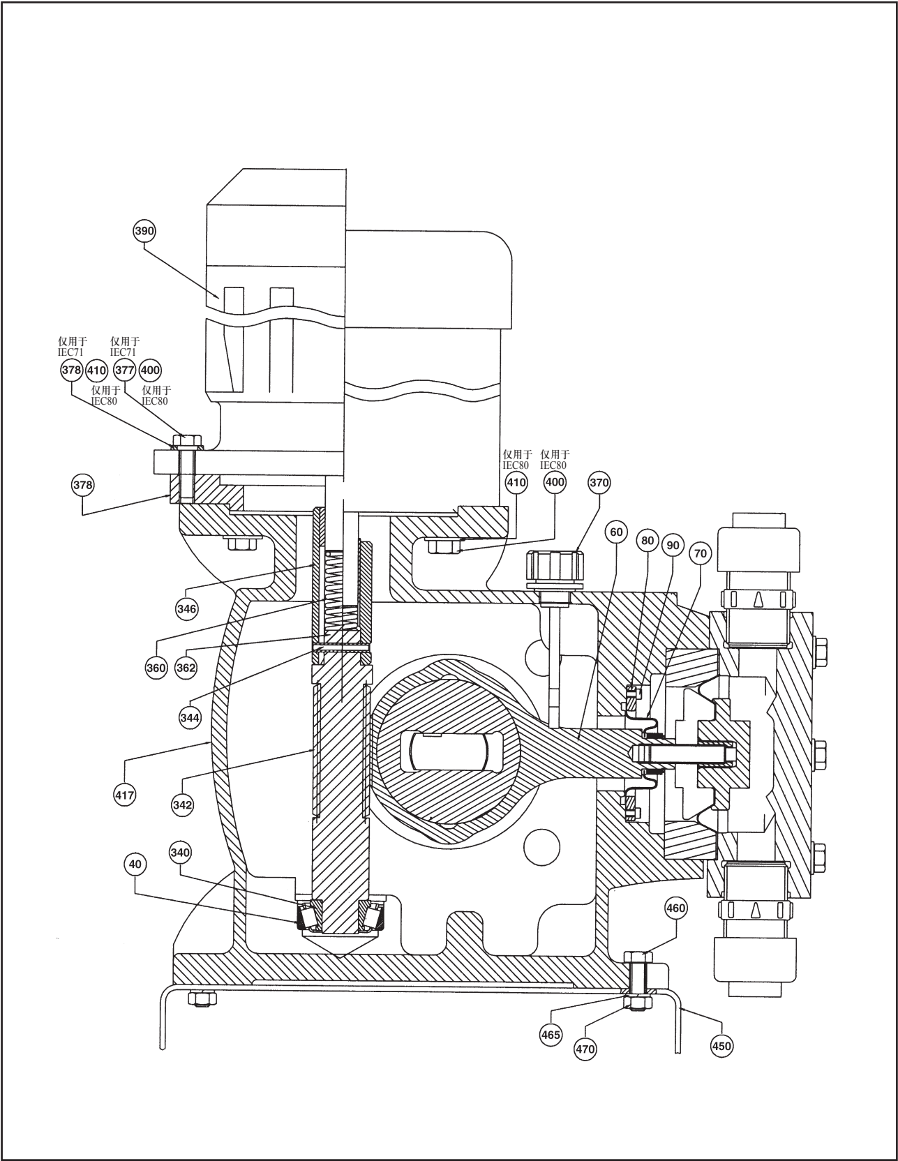
图6-1 GB系列基本部件——侧视图
