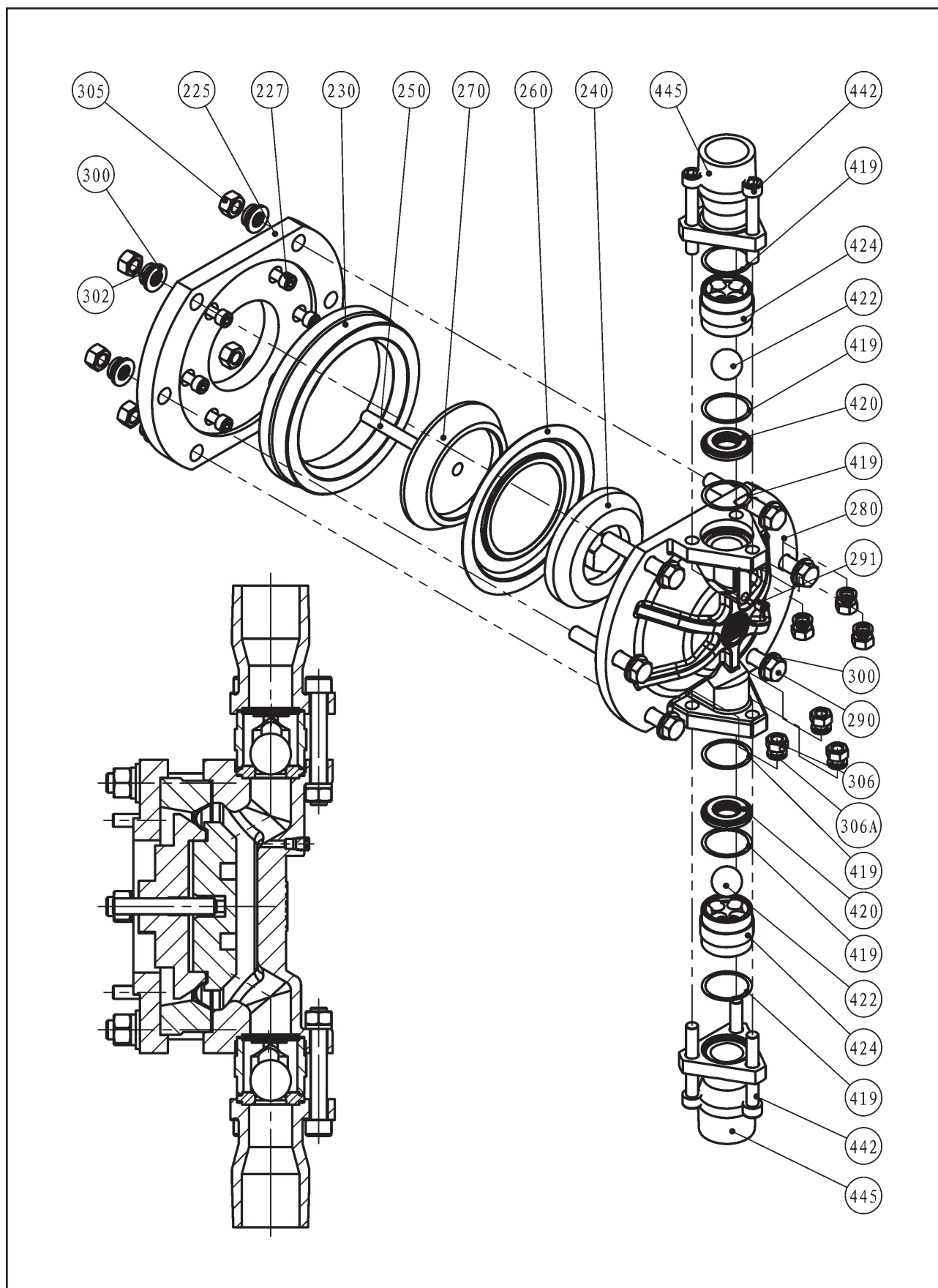
图6-15 GB1500不锈钢液力端
