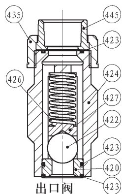
图6-8 GB0700~GB1200高粘度单向阀
