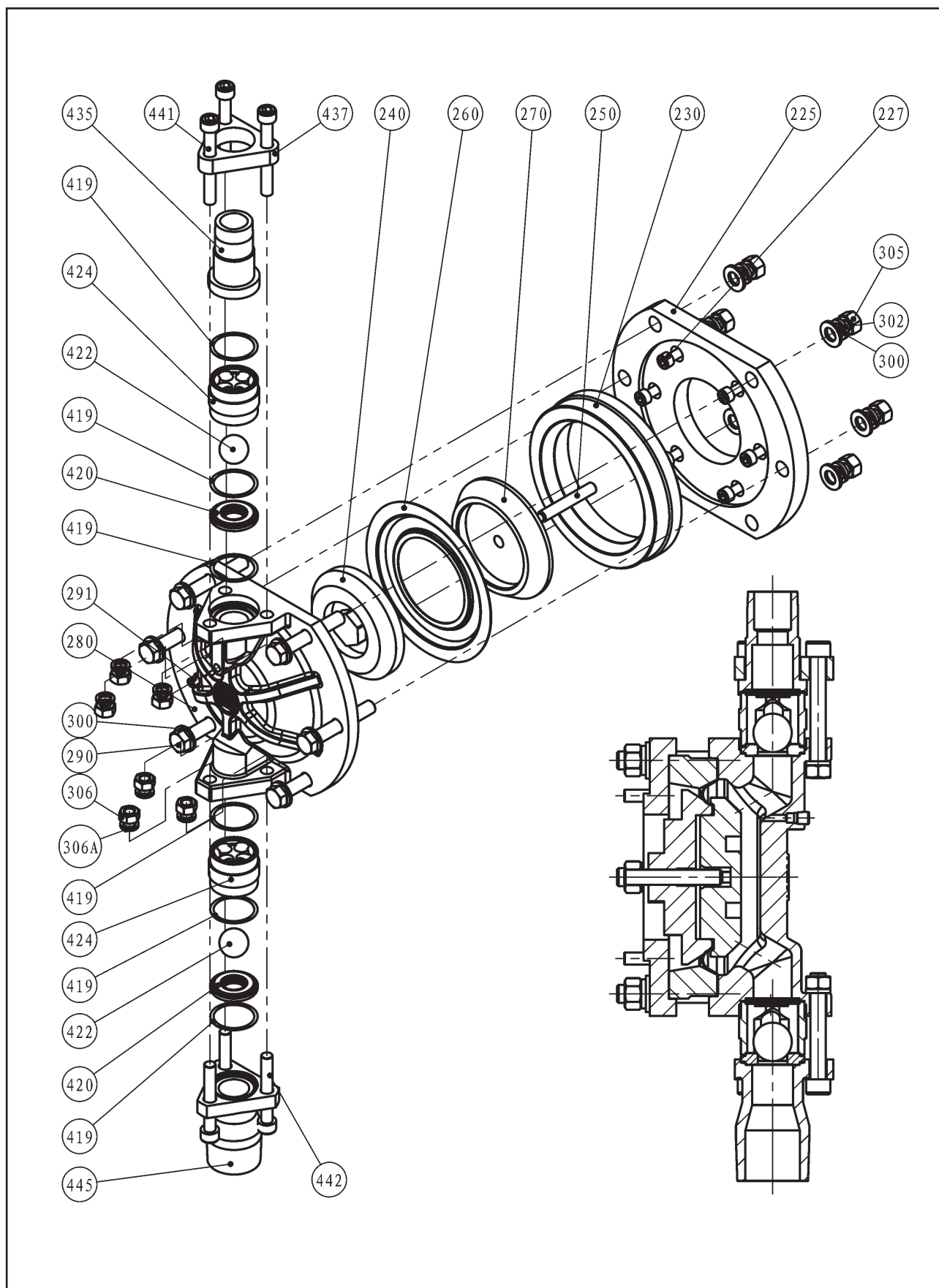
图6-14 GB0700~GB1200不锈钢液力端
