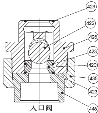
图6-9 GB1500塑料单向阀
