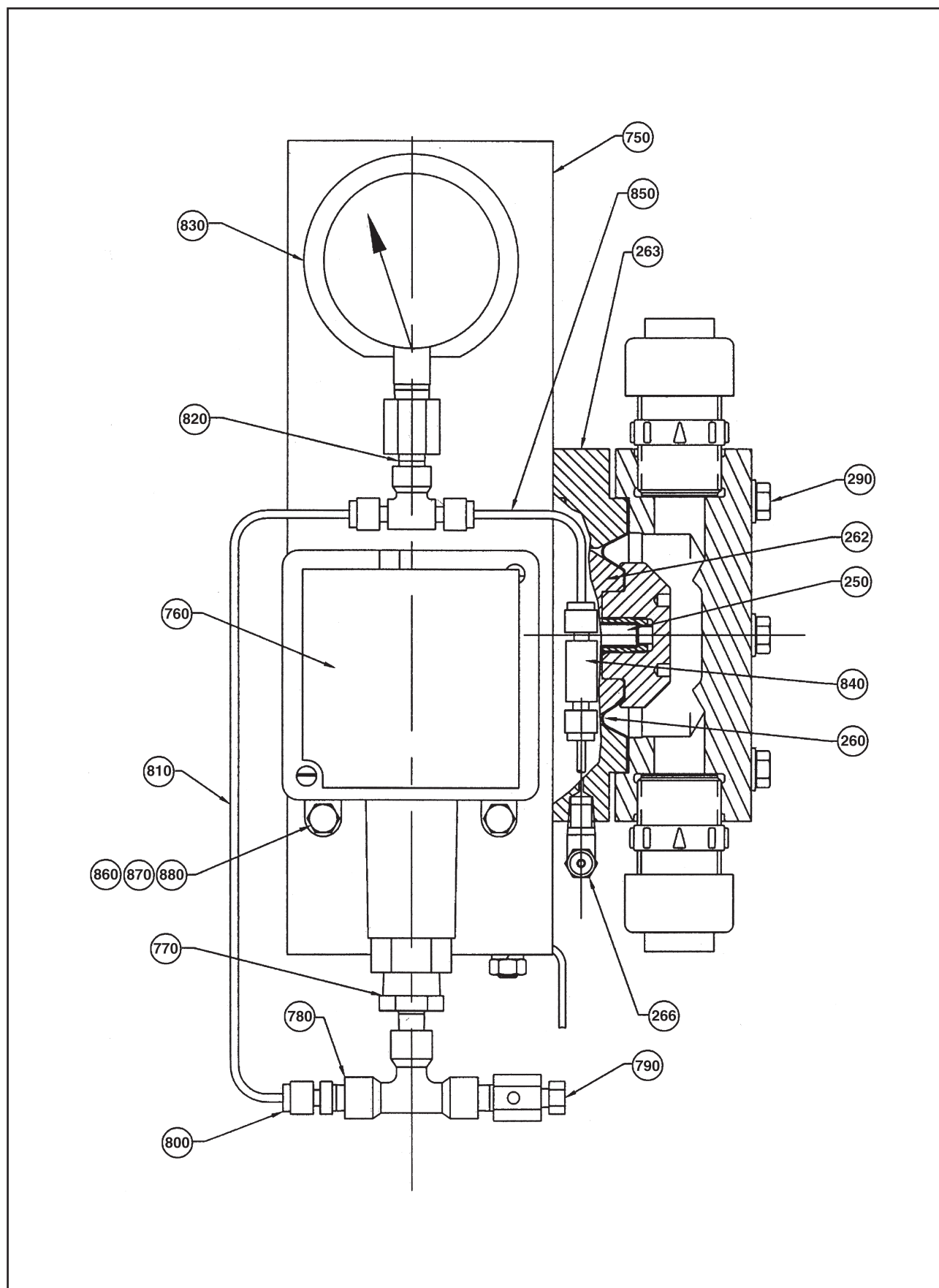
图6-18 泄漏检测，带压力表和压力开关（所有标准液力端）
