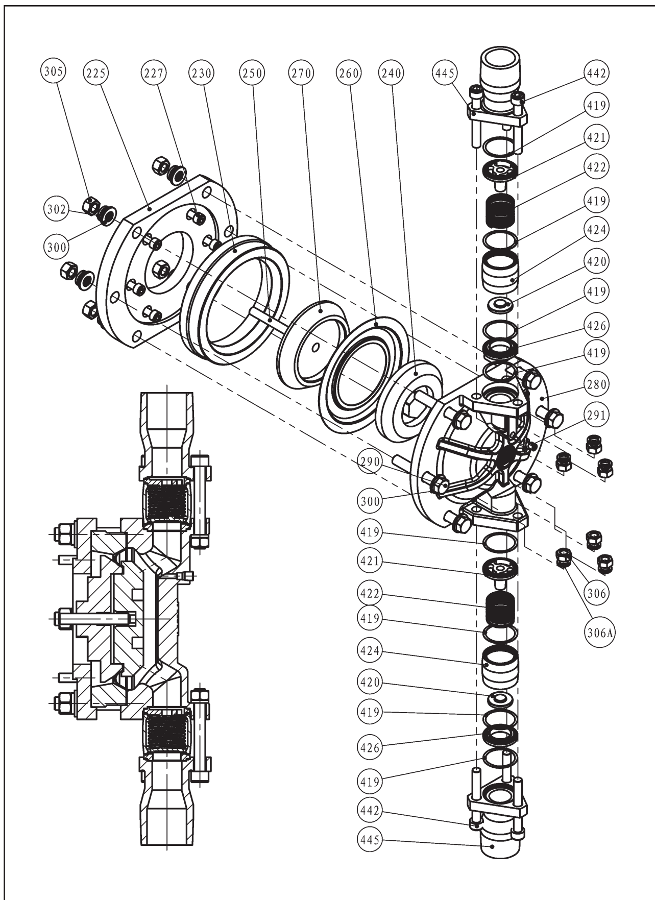
图6-16 GB1800 不锈钢液力端
