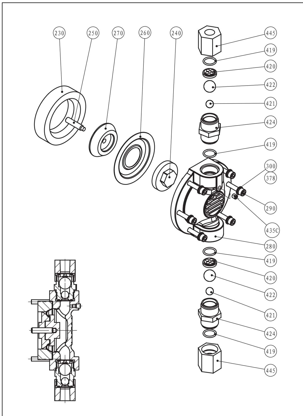
图6-12 GB0080~GB0450不锈钢液力端
