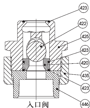
图6-7 GB0700~GB1200塑料单向阀
