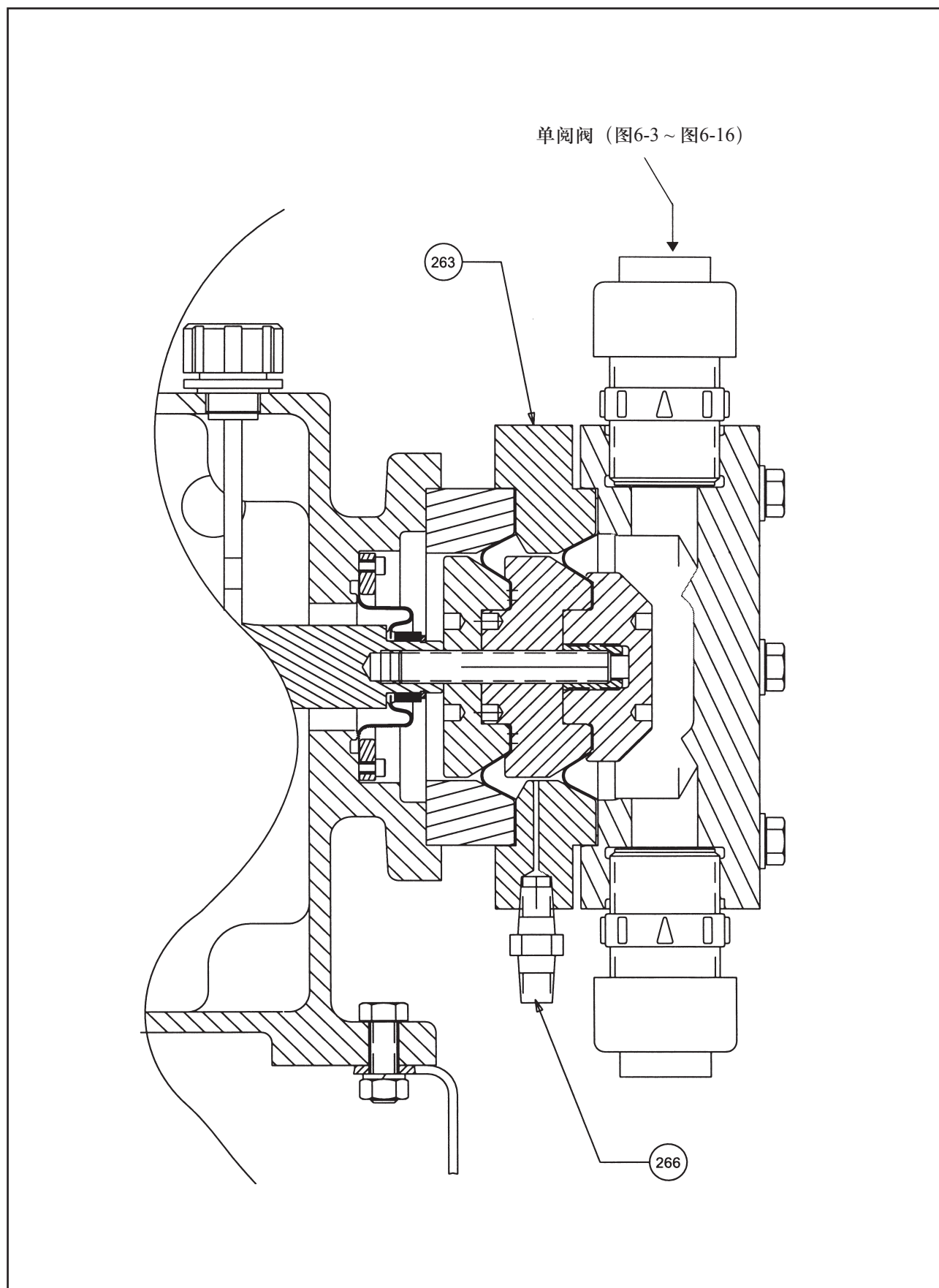
图6-17 双隔膜（所有标准液力端）
