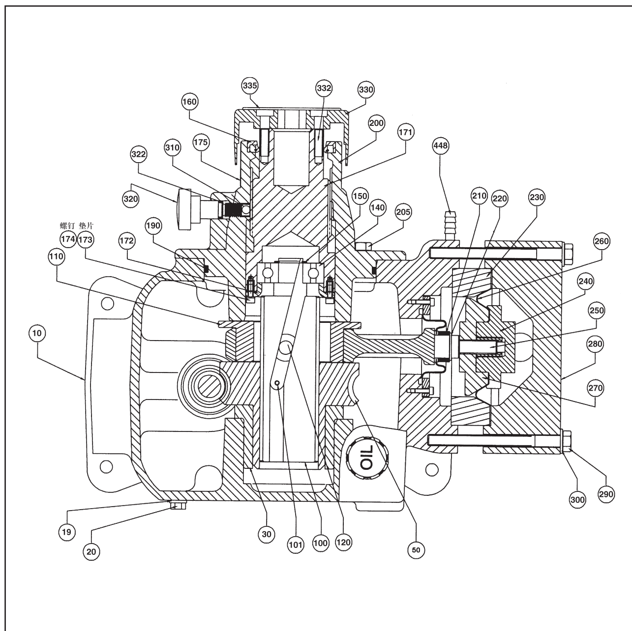
图6-2 GB系列基本部件——顶视图
