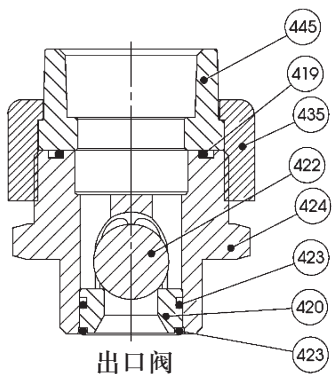
图6-9 GB1500塑料单向阀
