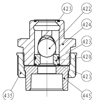
入口阀
